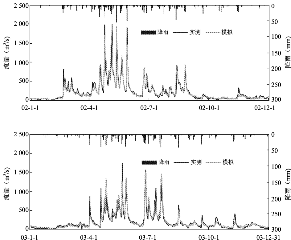
图 4 分布式 TOPMODEL 率定期(2002 年)与校验期(2003 年)模拟结果示意图
