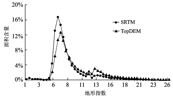
图 2 两种 DEM 数据计算得到的流域地形指数分布图 Fig.2 Distribution of Topographic Index Derived from SRTM and TOPDEM
