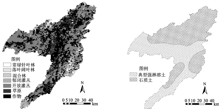
图 3 流域土地利用图与土壤图
