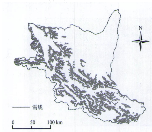
图 9 叶尔羌流域平均雪线(1979, 1990, 2000)
